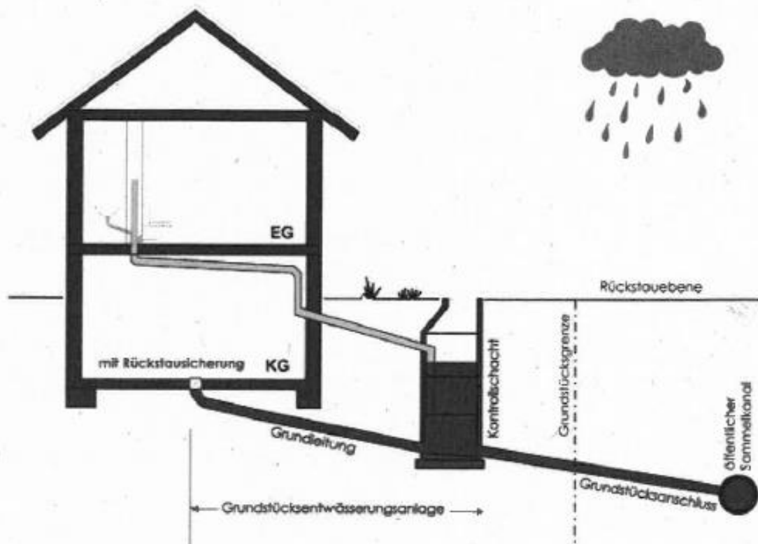
Abb.4 Grundstücksanschluss bei der Abwasserentsorgung (im Schnitt)
